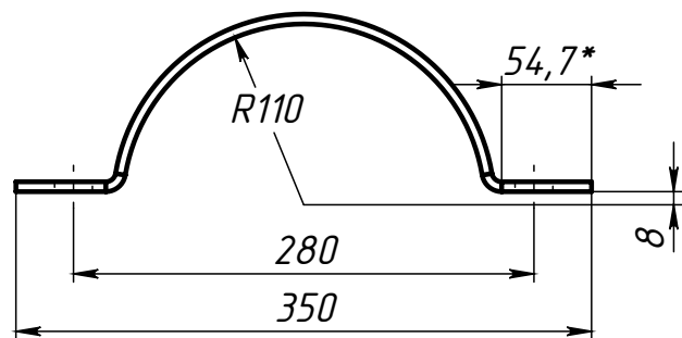
Поз.5 (Полухомут)
