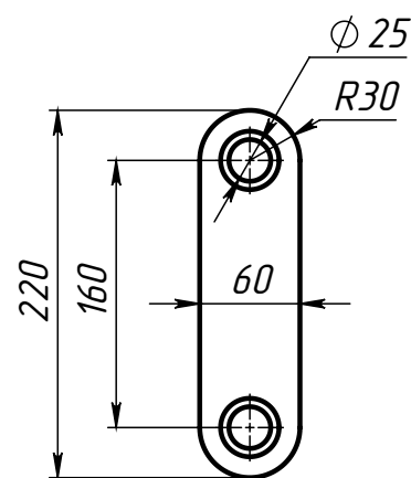
Поз.4 (Серьга)
