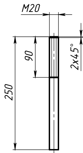
Поз.1 (Шпилька)
